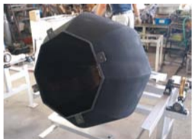
▲八角形のドラムを回転、かくはんしながらプロパンガスの火力で焙煎する。ドラム外周に特殊塗料を塗布した遠赤発生装置を装着している
